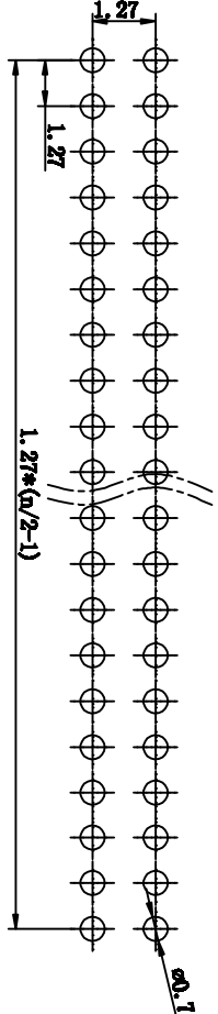
P.C.B Layout
