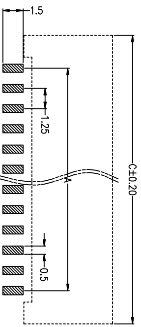
PCB 寸法 (PCB layout)
