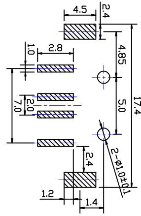
P.C.B Layout
