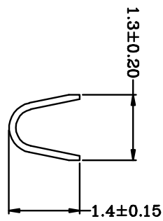
SEC:A-A
